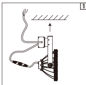
1. U字アームの内側から、壁にM10ボルトで固定します。
